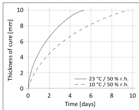
Schema 1: Uithardingssnelheid voor Sikaflex®-298 FC
